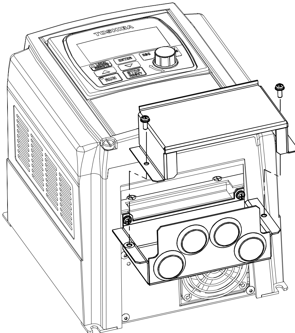
Figure 1. Conduit Extender Box.
