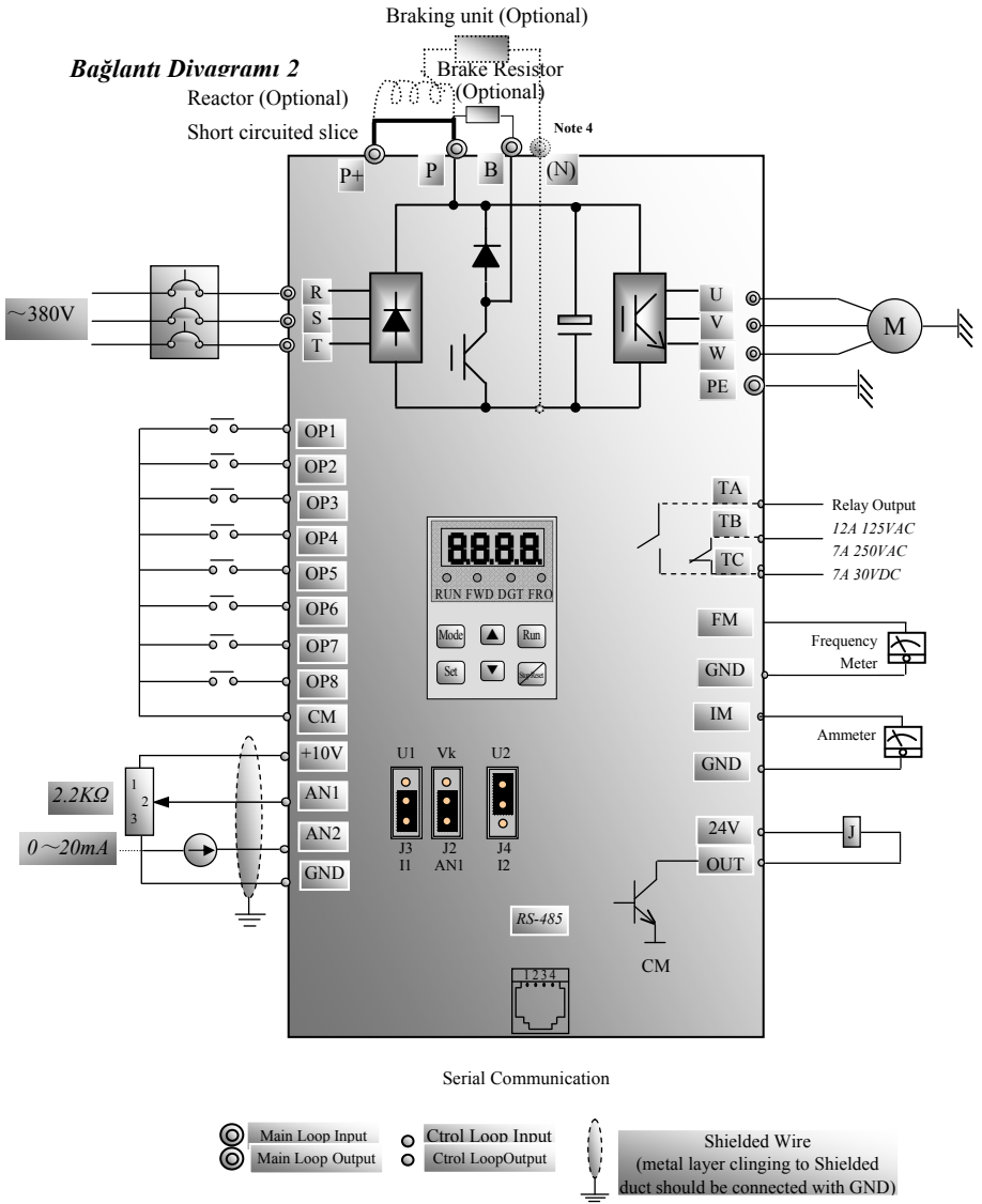
Fig 3-4 Trifaze Hız kontrol Cihazının Standart bağlantı Şeması
