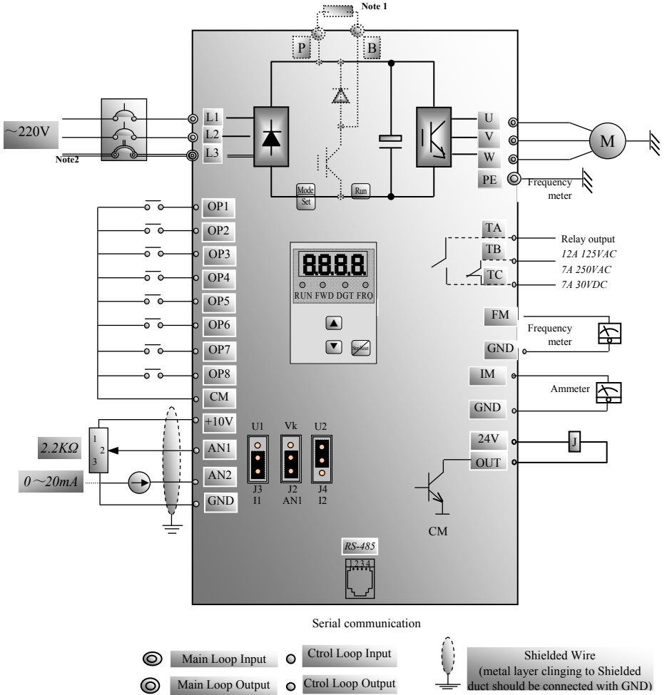
Fig 3-3 Monofaze Hız kontrol Cihazının Standart Kurulum Şeması
