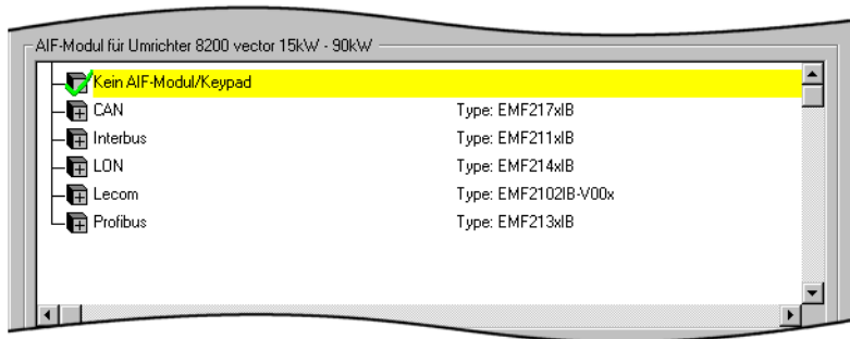
Abb. 4 Listenfeld AIF-Modul für ... im Dialogfeld AIF-Modul dem Grundgerät zuordnen
