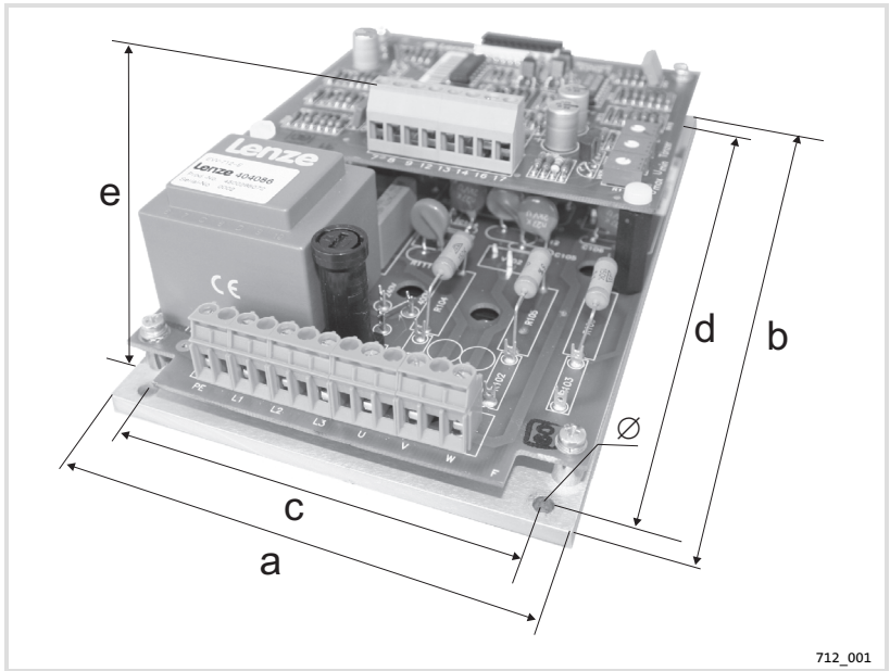
Fig. 1 Dimensions
