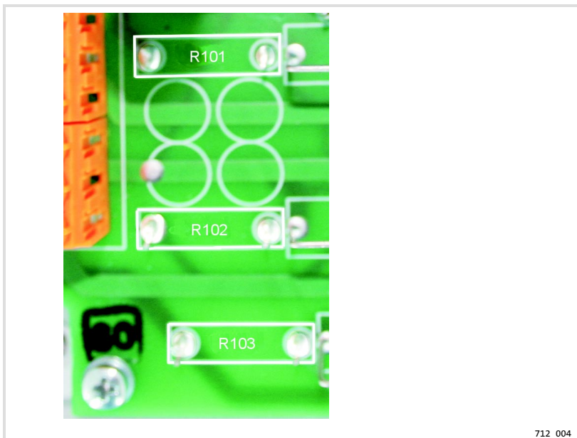
Abb. 5 Umstellung des Antriebsstellers 712 auf Netzanschluss 190 ... 265 V durch Einlöten von 220 k \Omega - Widerständen
