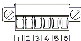
図 2.2 PROFIBUS 端子台
