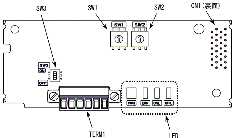
図 2.1 OPC-G1-PDP の外観
