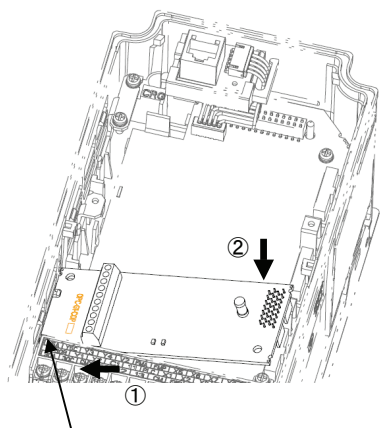
図 3.2 通信カードの取付け (A-port 取付け時)
