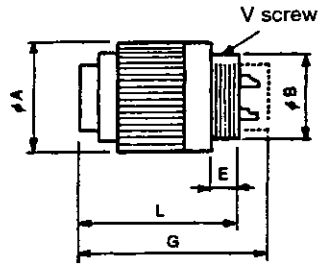
Plug JL04V-6A
