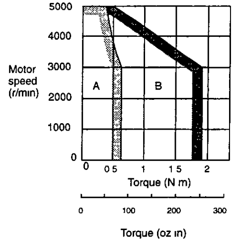
SGMAH-02B
