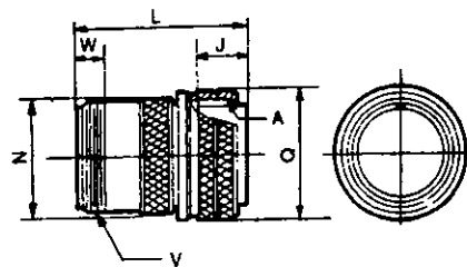
MS3106A Straight Plug Solid Shell
